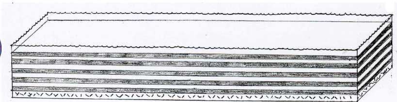
a. Pre-Pangea
