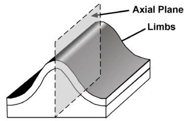
a. Symmetrical
