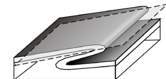
d. Recumbent
